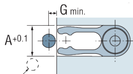
RITENSORE SGANCIATO
