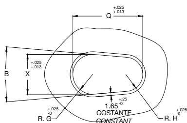
Dimensioni per foro inserimento True-Fit Hole dimensions for true-fit inserts
